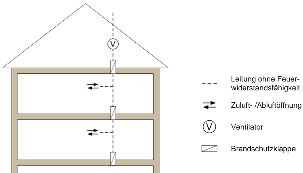
Bild 2.1: Schottlösung
