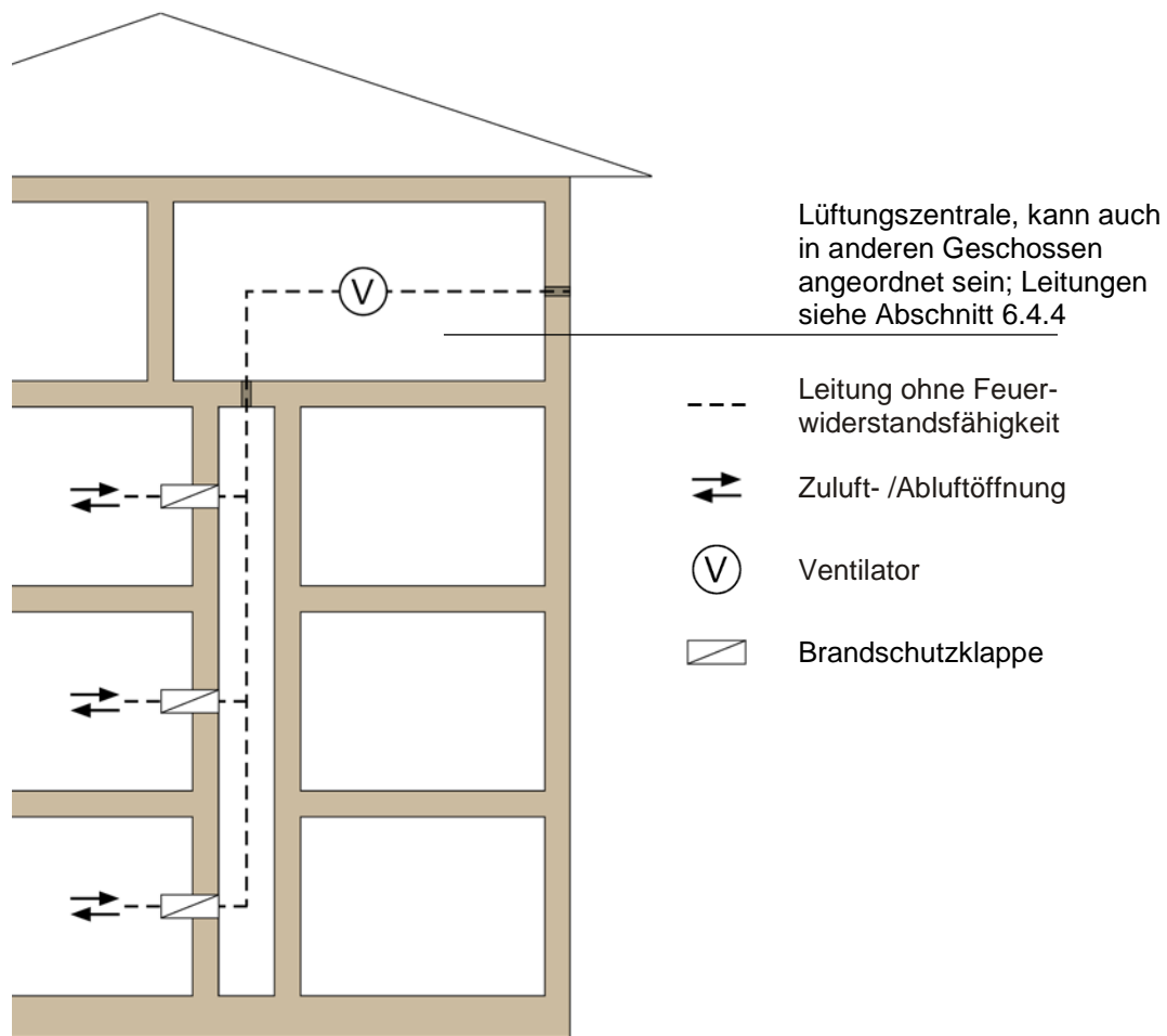
Bild 1.2: Schachtlösung
